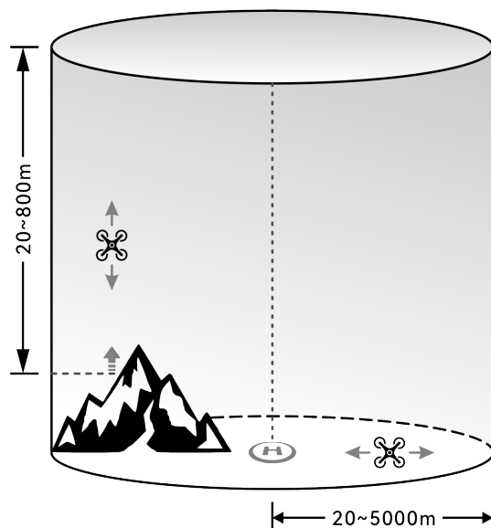
图 2-5 限高限远示意图
