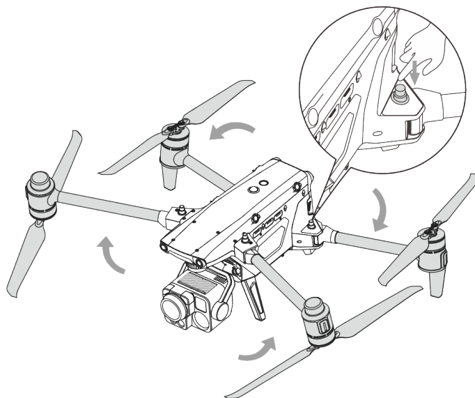
图 3-6 机臂折叠示意图
