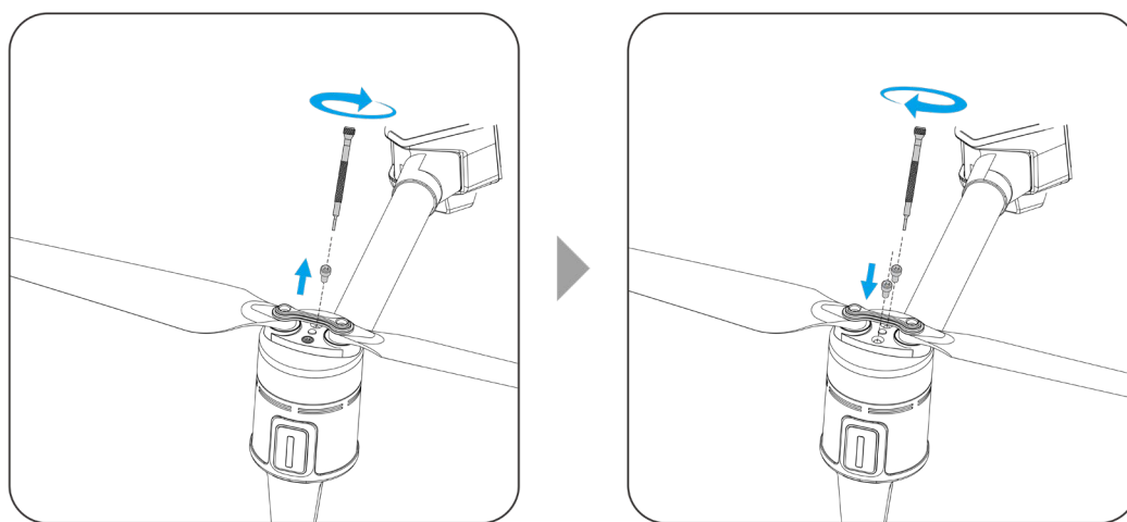
图 3-8 螺旋桨安装示意图
