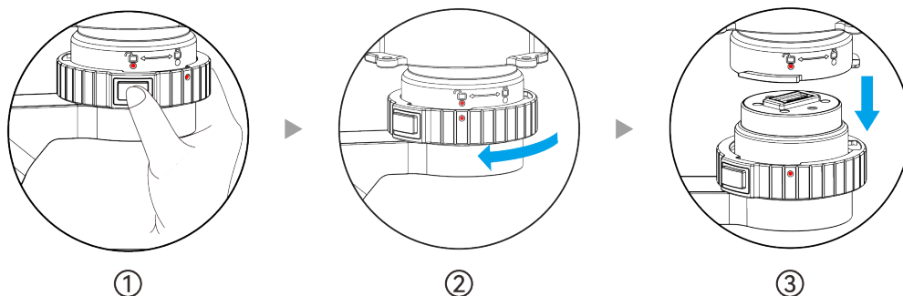
图 3-16 从无人机上取下云台
