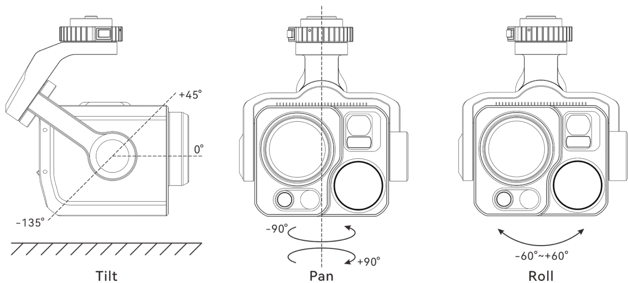
图 3-14 云台结构设计范围（图示为慧眼 L35T 云台）
