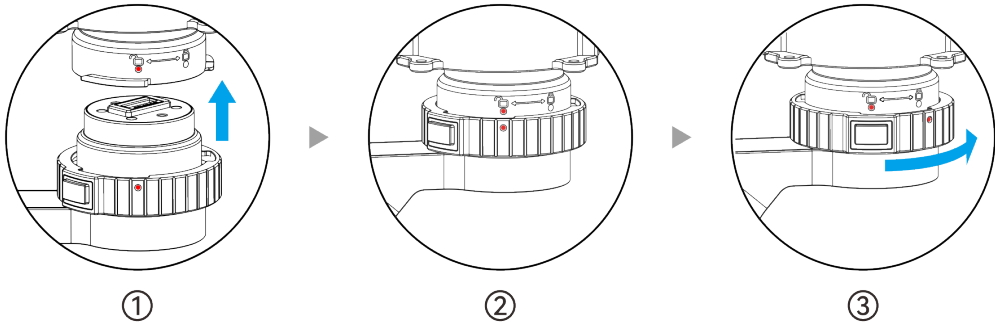
图 3-15 为无人机安装云台
