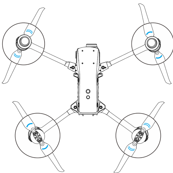
图 3-7 无人机螺旋桨安装布局（丝印标识均朝向机身顶部）
