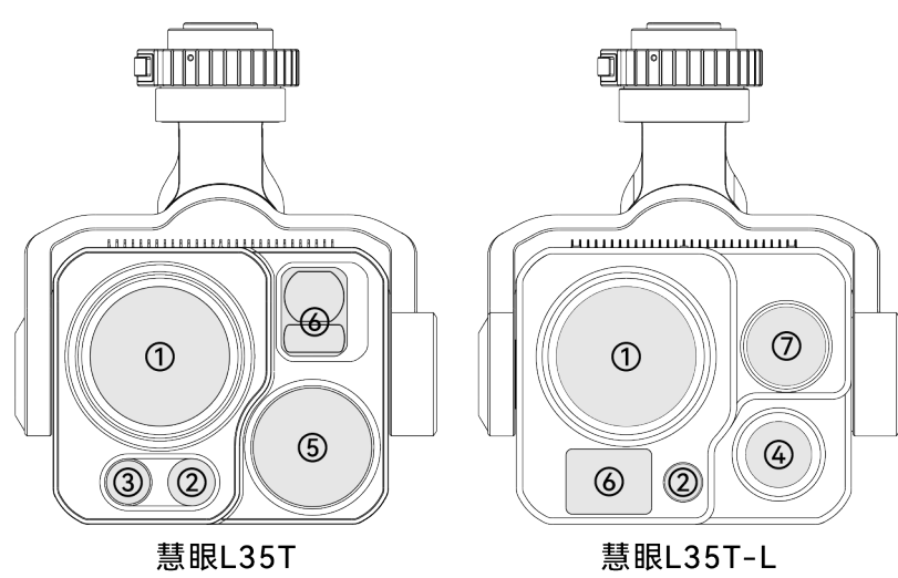
图 3-12 云台相机布局
