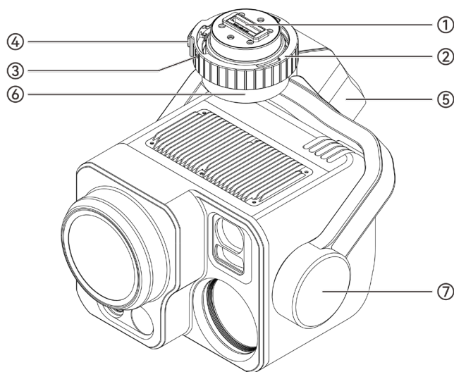
图 3-13 云台结构
